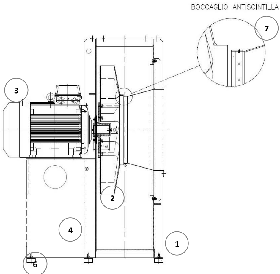
Slika 6. Centrifugalni ventilator – IZRAVNI prienos – Pogled s boka (Tablica A)
